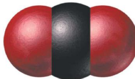
CO 2
