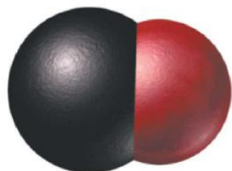
CO
